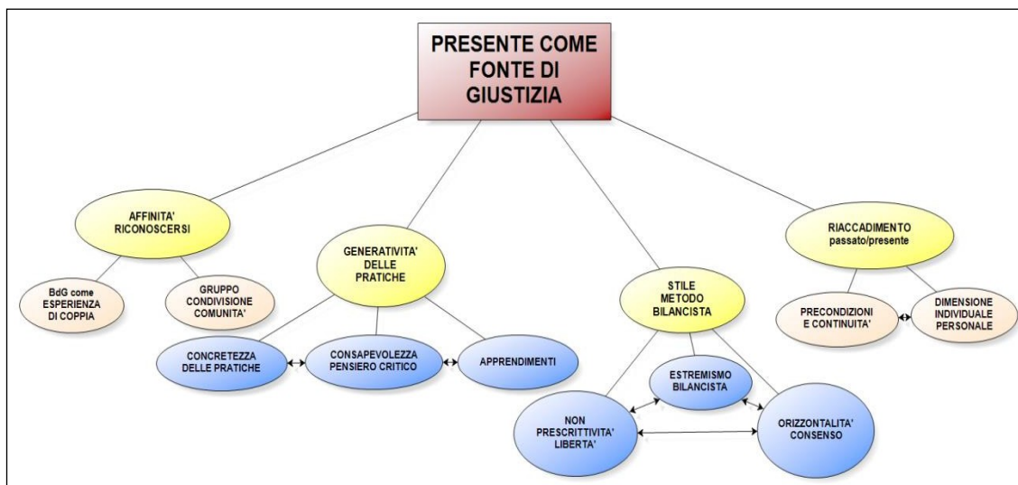
Figura 7 Raffigurazione teoria
