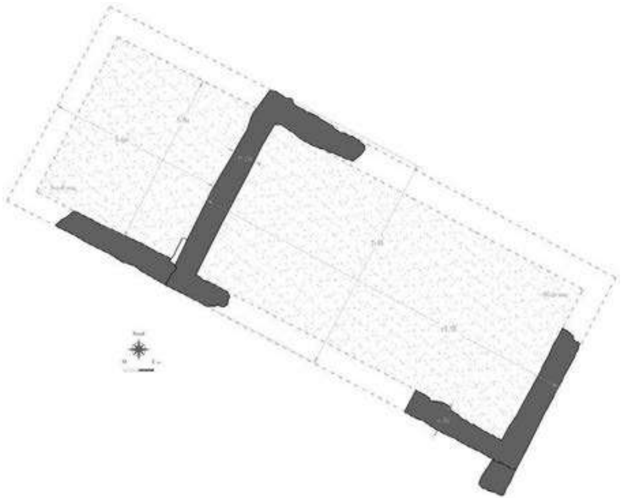
Figura 7. Planimetria del palazzo del castello.
