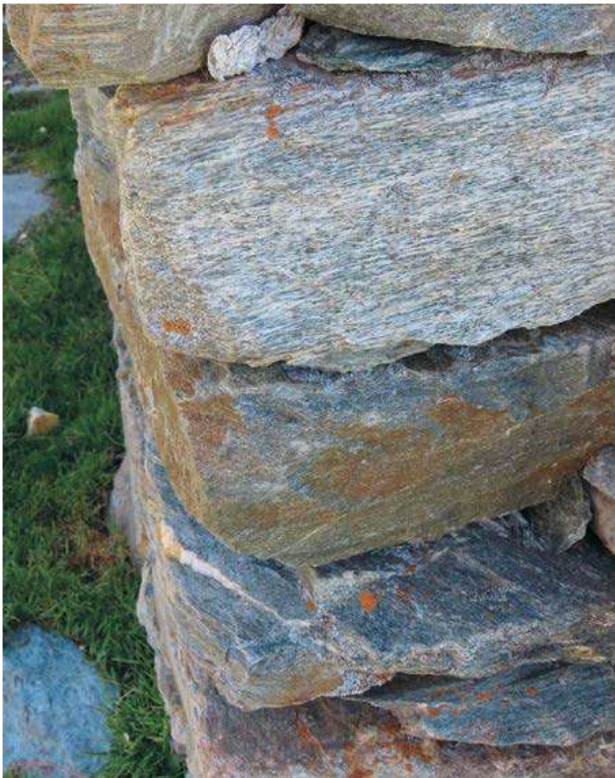
Figura 1. Elementi da muratura di una costruzione rurale ad uso abitativo. Si noti la varietà litologica, ogni elemento infatti è costituito da rocce diverse: serpentinite, anfibolite, orto-gneiss. Il fattore comune è l'orientazione planare prevalente che guida lo spacco naturale lungo le due facce parallele al suolo e che facilita l'operazione di impilamento degli elementi e di costruzione della muratura.
