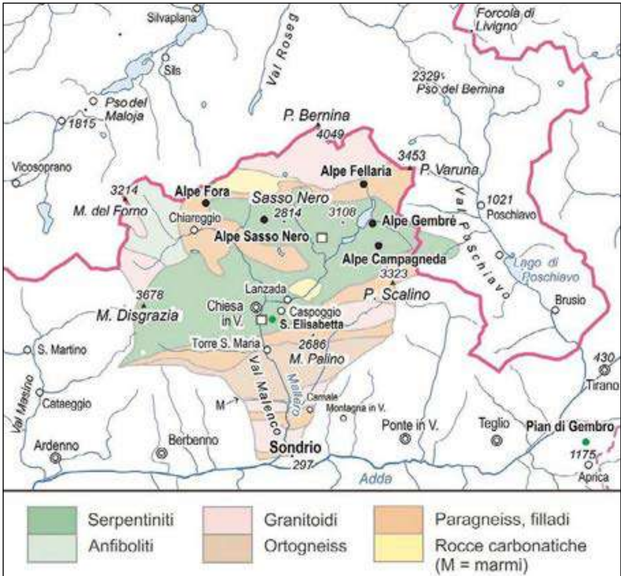
Figura 2. Carta litologica schematica della Valmalenco in base a Montrasio e Trommsdorff (2004) armonizzata in base alle distinzioni geoecologiche presentate in Tabella 1. L'area di affioramento della serpentinite è stata estesa oltre il bacino idrografico (base cartografica: Carta geografica vettoriale della Svizzera 1:500.000, Ufficio federale di topografia swisstopo).
