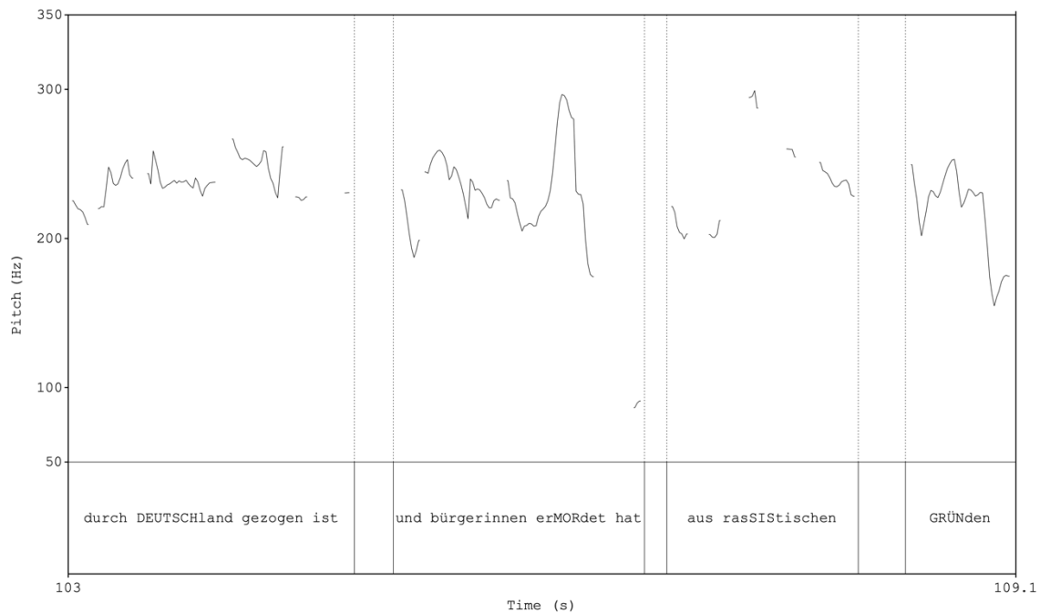
Figura 9 Grafico Praat dei ss. 04–09 in (63)
