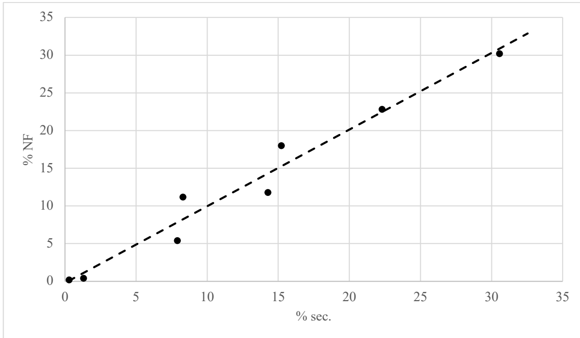
Figura 14 Dispersione lineare della durata complessiva dei discorsi in secondi (% sec.) e della percentuale di NF realizzati complessivamente (% NF) per gruppo.
