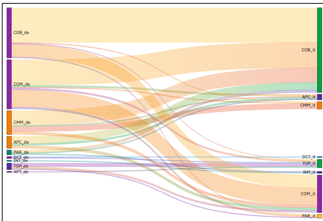
Figura 17 Flussi dalle unità prosodiche originali (sinistra) a quelle in traduzione (destra).
