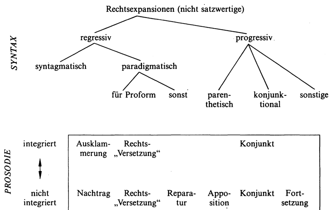
Figura 1 Caratteristiche sintattico-prosodiche delle espansioni a destra senza nuovo verbo in Auer (1991: 144–145).
