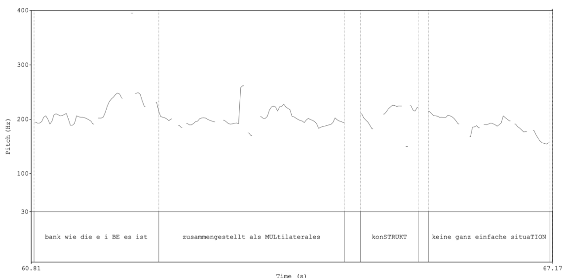
Figura 11 Grafico Praat ss. 03-08 in (68)
