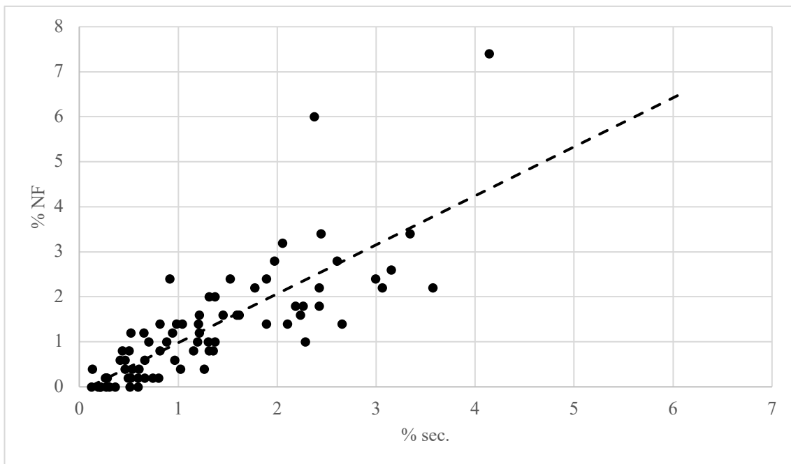
Figura 13 Dispersione lineare della durata complessiva dei discorsi in secondi in percentuale (% sec.) sui NF realizzati complessivamente in percentuale (% NF) per parlante.
