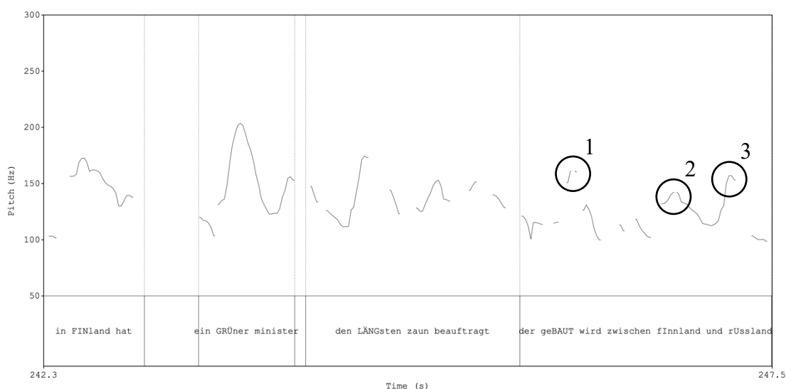
Figura 12 Grafico Praat di (69)
