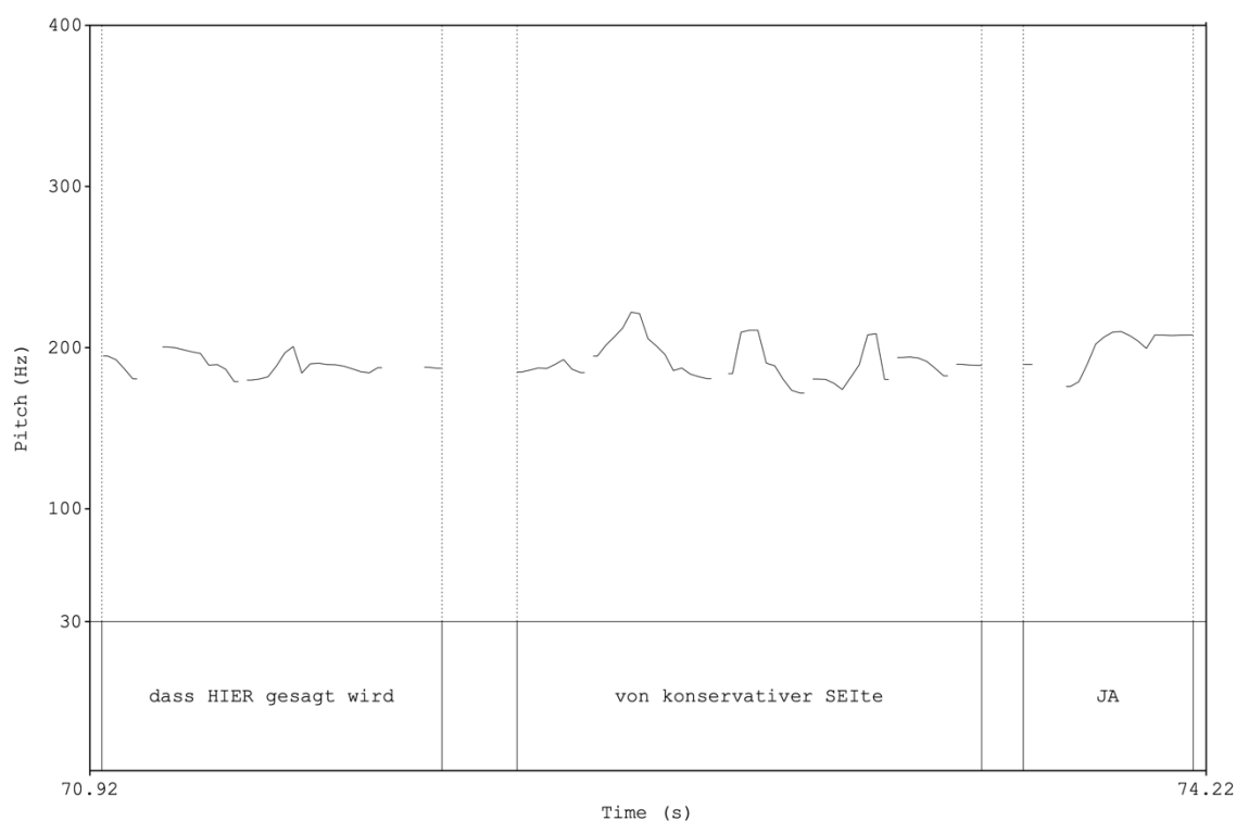
Figura 10 Grafico Praat dei segmenti 05-09 in (67)
