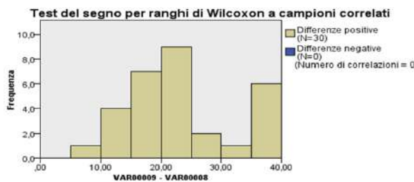
Fig. 5: Test del segno per ranghi di Wilcoxon e campioni correlati
