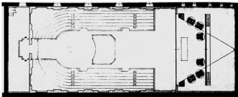
Fig. 3. Ipotesi di ricostruzione in pianta del teatro Mediceo degli Uffizi, versione 1589 (Annamaria Testaverde-Saverio Balli 1990. Da Testaverde 1991, p. 28, fig. 7).
